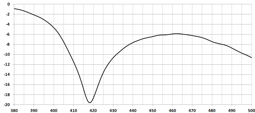
Rückflußdämpfung / Return loss
