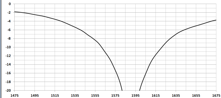
Rückflusdämpfung / Return loss
