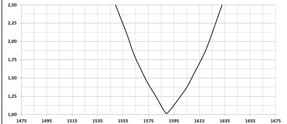
VSWR
